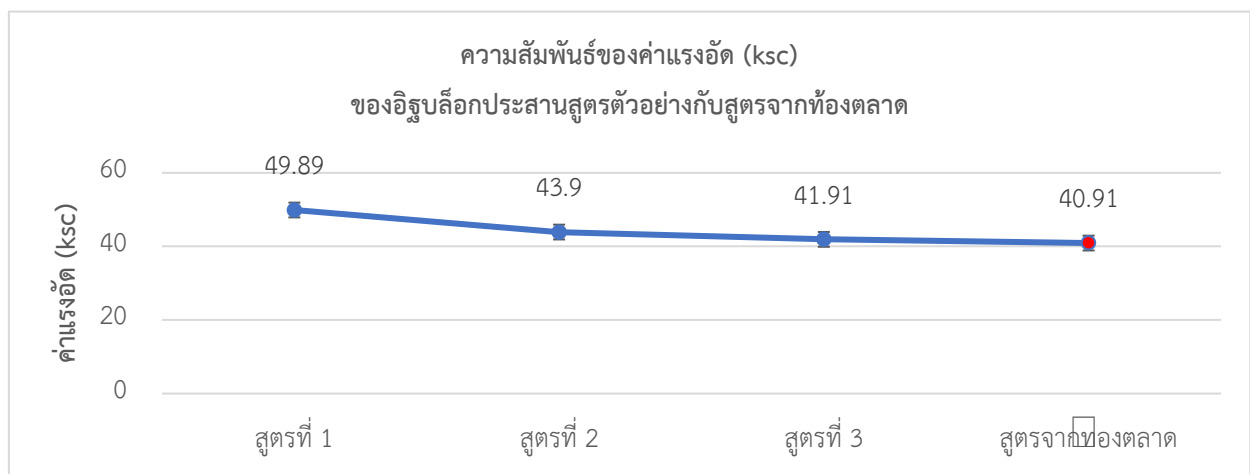
ภาพที่ 7 แสดงความสัมพันธ์ของค่าแรงอัด (ksc) ของอิฐบล็อกประสานสูตรตัวอย่างกับสูตรจากท้องตลาด
