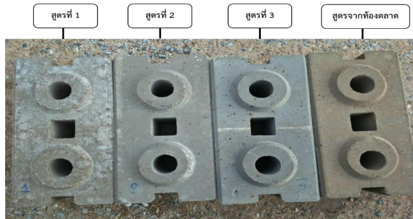
ภาพที่ 4 อิฐบล็อกประสานที่มีส่วนผสมของเถ้ากะลามะพร้าวแต่ละสูตรกับอิฐบล็อกจากท้องตลาด
